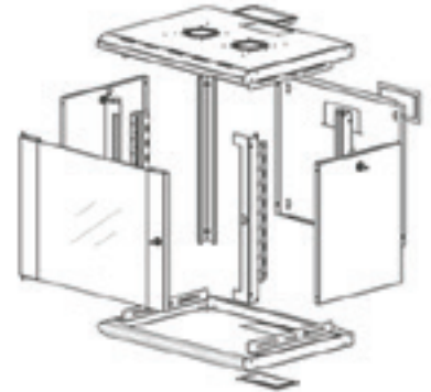
PATLATILMIŞ GÖRÜNÜM
