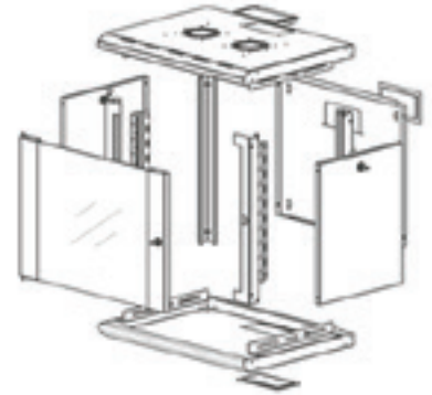
PATLATILMIŞ GÖRÜNÜM
